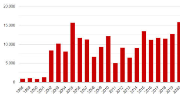
Figura 1 - Série histórica do total de focos ativos detectados pelo satélite de referência, no período de 1998 até 13/10/2020.
